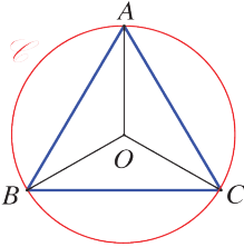
مثلث متساوي الساقين
